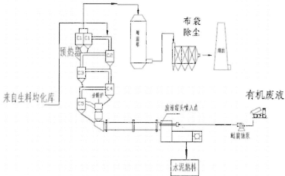
图 4.9-3 有机废液预处理及输送投料工艺流程图
