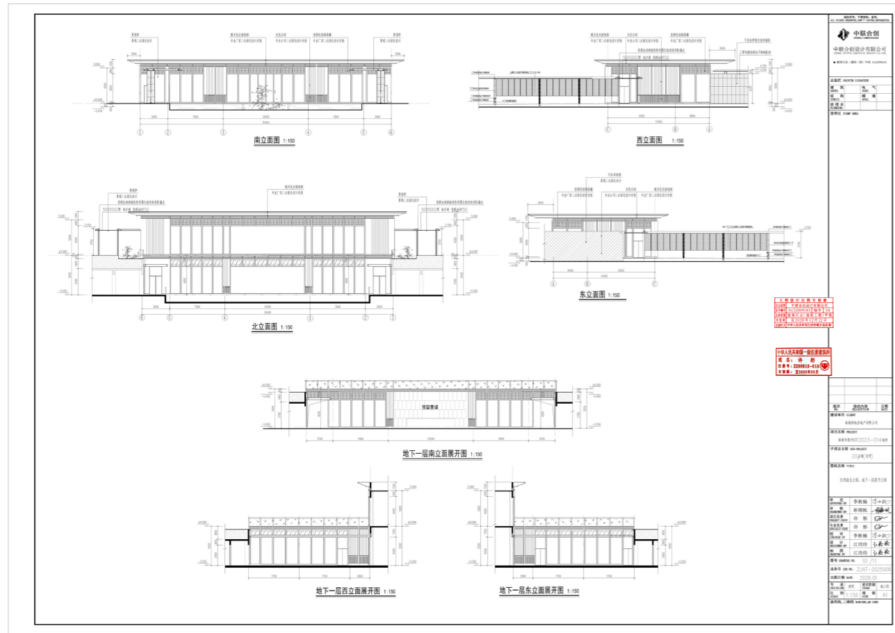
20#楼立面图
