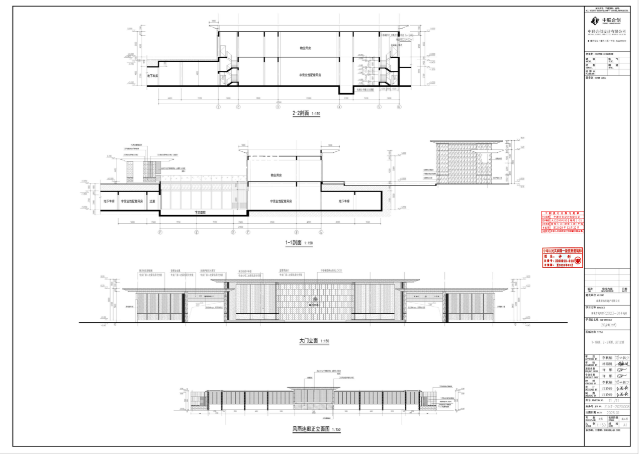
20#楼剖面图
