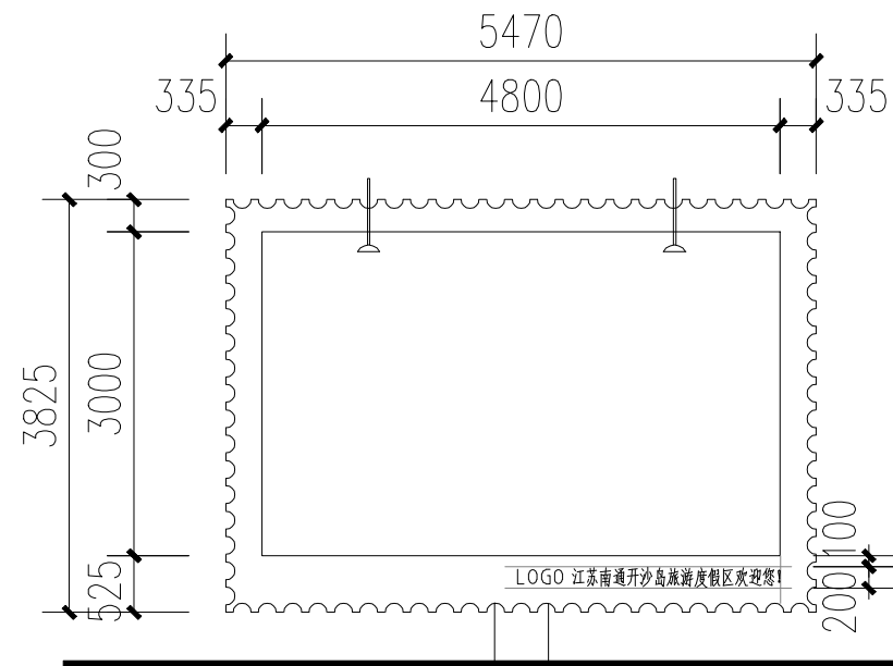
规格一正立面图
