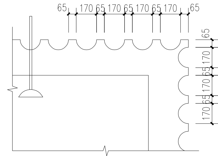
齿口尺寸
