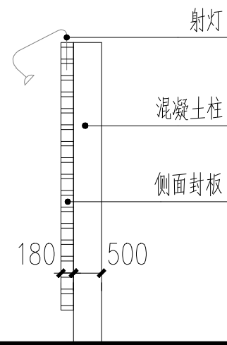
规格一侧立面图
