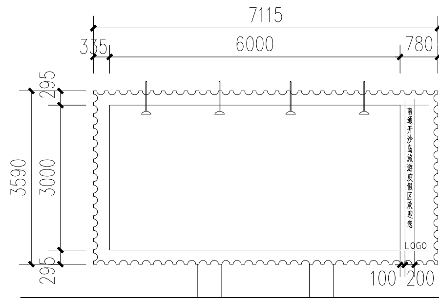
规格二正立面图
