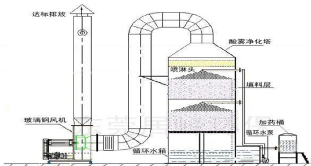
图 4-3 废气处理工艺流程图
