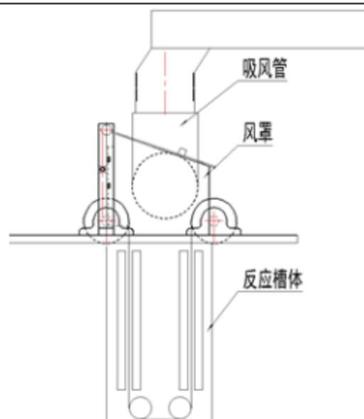
图 4-2 生产线盖式集气罩示意图
