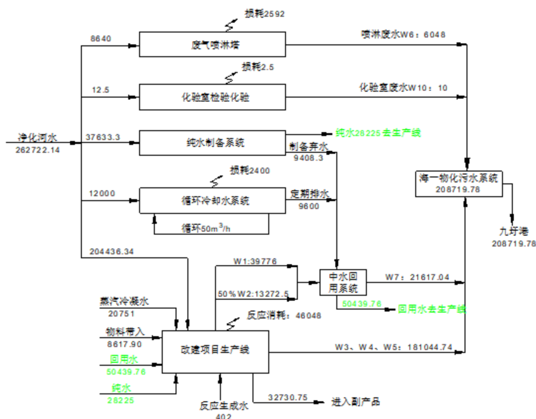
图 2-3 本项目水平衡图 (t/a)
