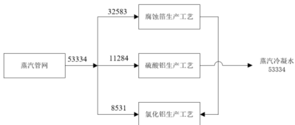
图 2-2 改建后全厂蒸汽平衡 (t/a)
