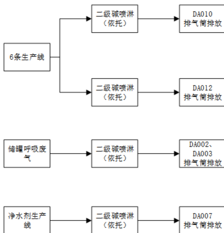
图 4-1 废气处理流向示意图
