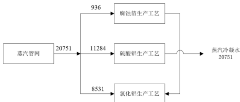
图 2-1 项目蒸汽平衡 (t/a)
