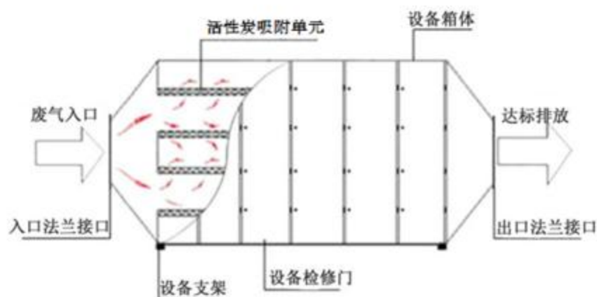
图 4-2 活性炭装置原理示意图
