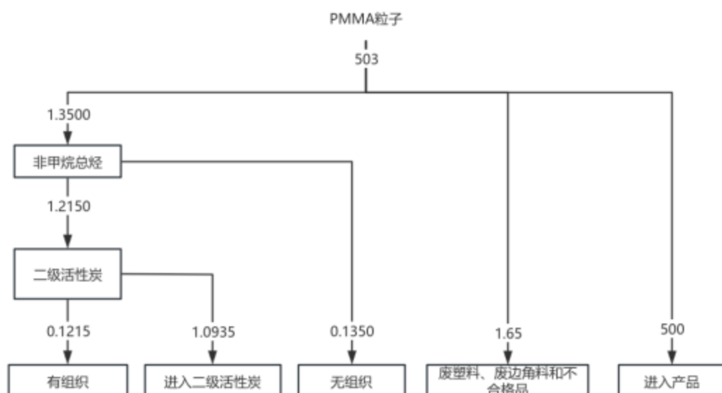
图 2-2 物料平衡图（单位：t/a）
